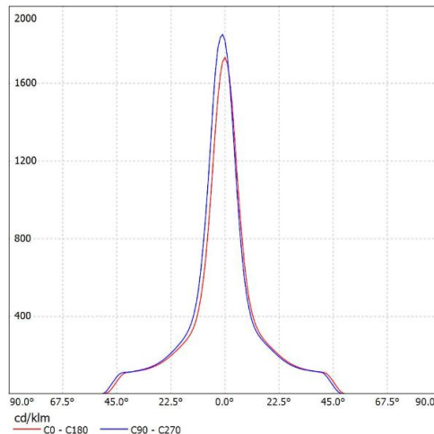
SL-04413A K:4.84cd/lm,LED:CXA1304
