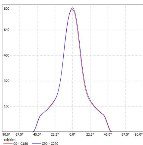
SL-04425A K:3.06cd/lm,LED:CXM-6
