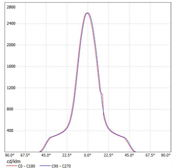
SL-04425B K:2.69cd/lm,LED:G4-10
