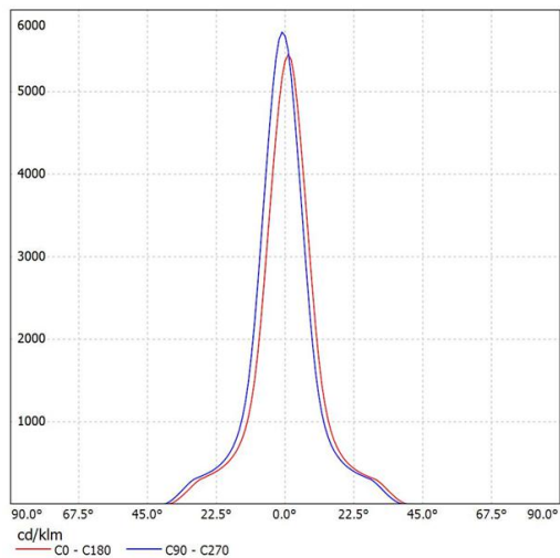
SL-05015A K:7.35cd/lm,LED:1507
