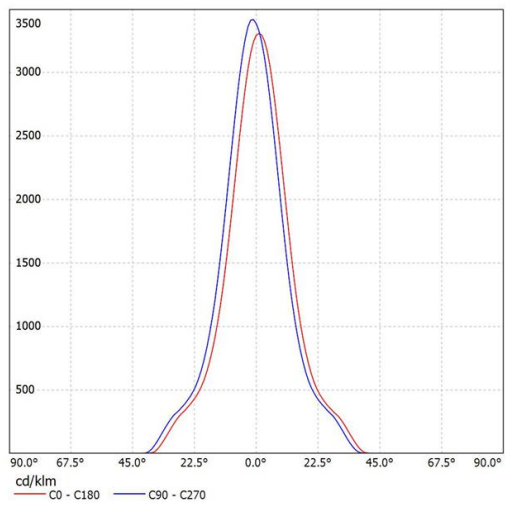
SL-05024A K:4.35cd/lm,LED:1507
