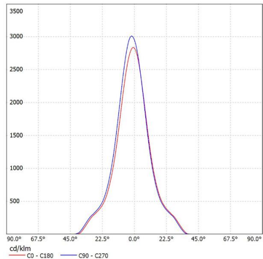
SL-05024A K:4.33cd/lm,LED:CXM-9
