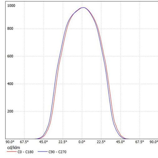
SL-05060D K:1.24cd/lm,LED:1507
