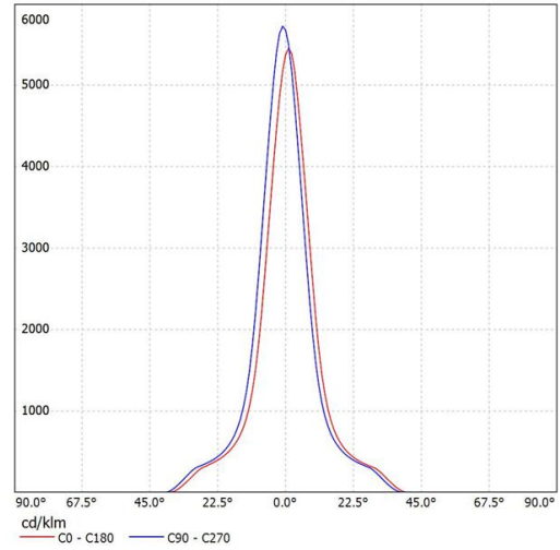
SL-05015D K:7.35cd/lm,LED:1507
